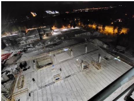
A-lohkon onteloasennuksia
