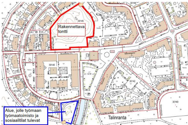
Työmaatoimiston ja työmaan sosiaalitilojen sijoitus
